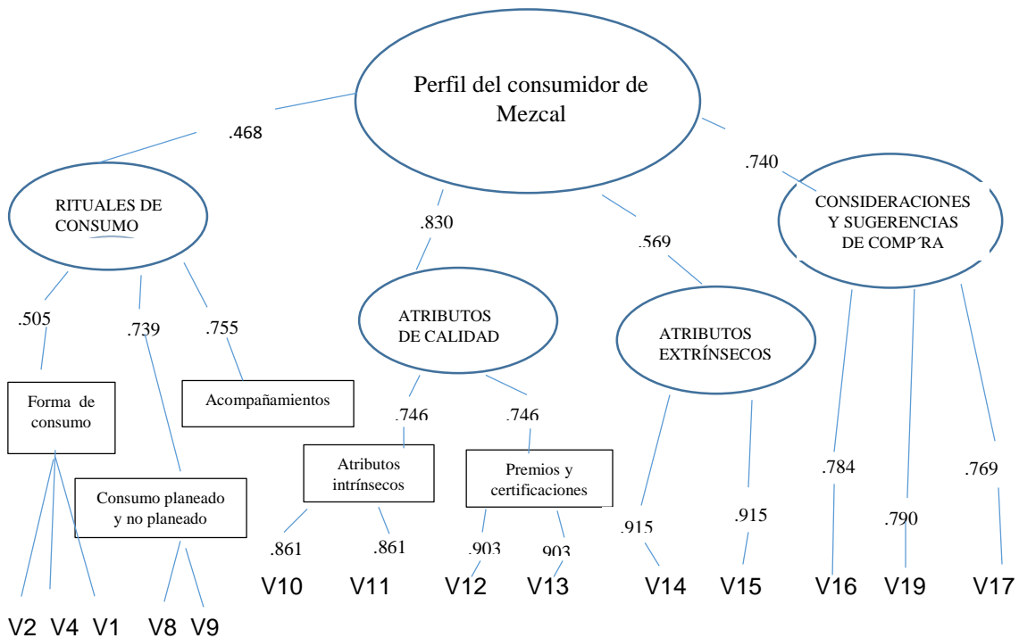
Figura 2. Ecuación estructural
